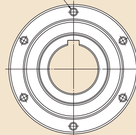
Фаски на торцевых поверхностях отверстия
