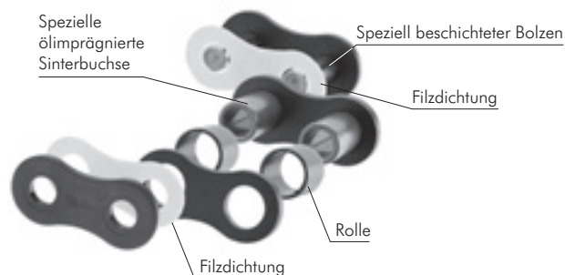
Abb. 11 Grundkonstruktion
