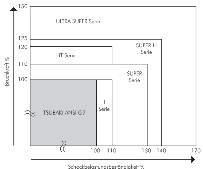
Abb. 16 Vergleich der Zugfestigkeit / Stoßfestigkeit
