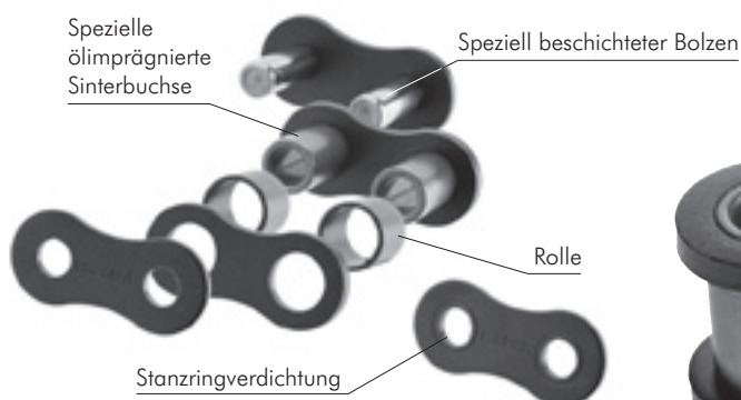
Abb. 10 Grundkonstruktion
