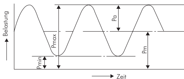
Abb. 4 Zusammenfassung für sich wiederholende Belastungskräfte
