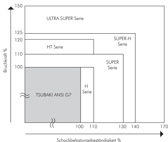
Abb. 16 Vergleich der Zugfestigkeit / Stoßfestigkeit
