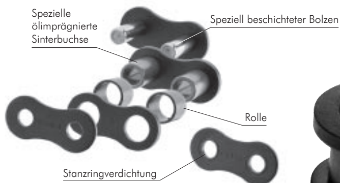
Abb. 14 Grundkonstruktion
