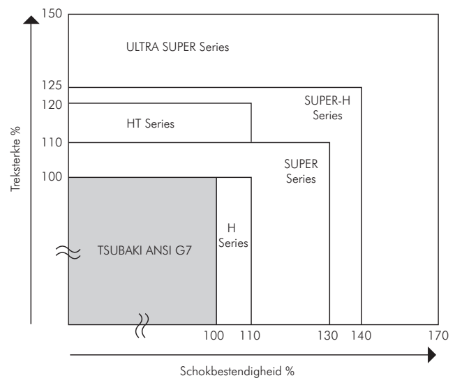
Fig. 16 Vergelijking treksterkte / schokbestendigheid
