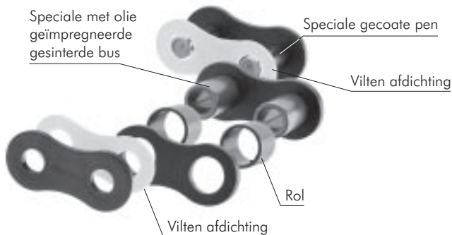
Fig. 11 Basisopbouw
