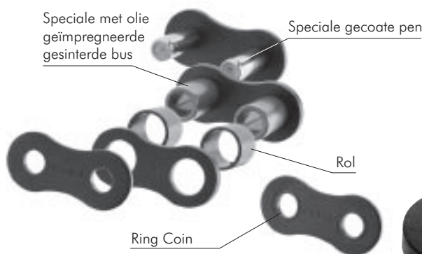
Fig. 14 Basisopbouw
