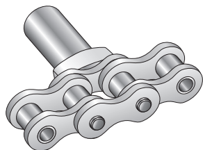
Fig. 15 : Tous les axes débordants (d'un côté)
