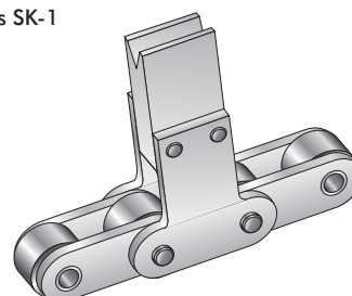
Fig. 14 : Attache SK avec bloc en V
