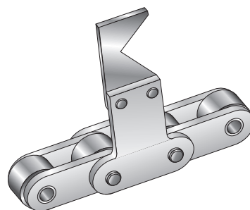
Fig. 12 SA meenemer met haak
