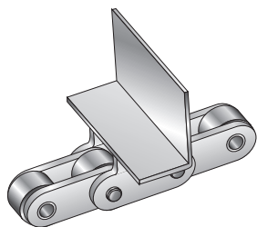
Fig. 10 K meenemer met hoeklijn
