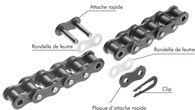
Fig. 11 Comment fermer la chaîne X-LAMBDA ASA
