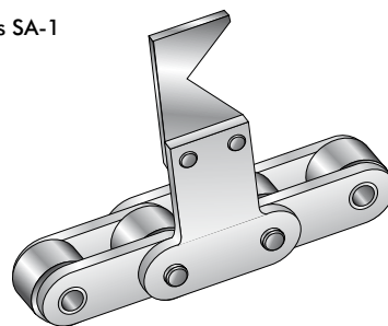
Fig. 21 Attache SA-2 avec crochet
