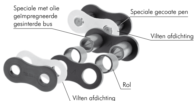
Fig. 10 Basisopbouw
